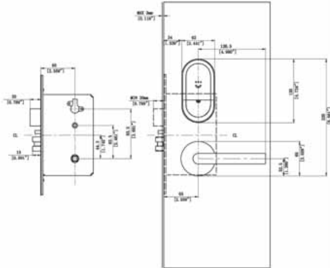
EURO lockcase
